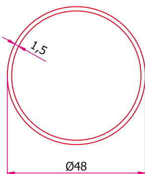
Armătură R508/15 Greutate: 1,72 kg/m Rinforzo: R508/15 Peso: 1,72 kg/m Merevítés: R508/15 Súly: 1,72 kg/m
