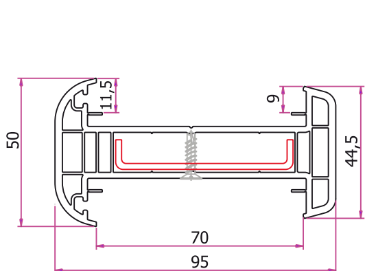
Profil de dilatare TP-6307 Profilo espansione TP-6307 Dilatációs profil TP-6307
