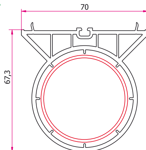
Cuplaj tubular TP-6305 Tubolare di aggancio TP-6305 Csősoroló TP-6305
