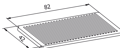
Cală plană g=1, 2, 3,mm TP-5628 Spessore per vetrata g=1, 2, 3,mm TP-5628 üvegezőék g=1, 2, 3,mm TP-5628
