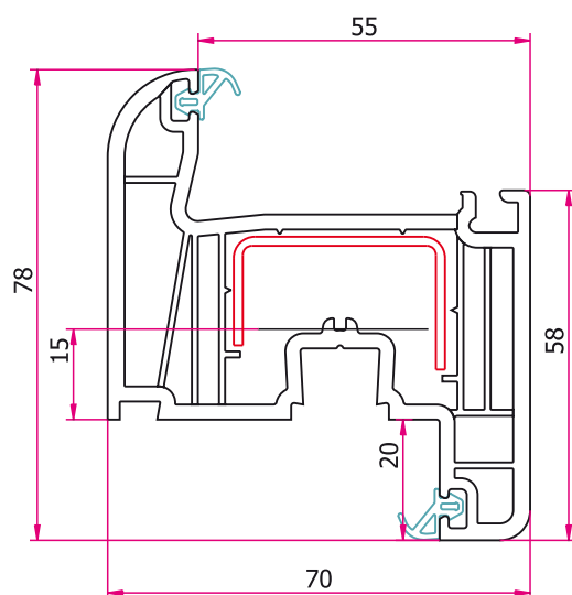
Cercevea TP6102 - standard Cercevea TP6102 - Eco Anta finestra TP6102 - standard Anta finestra TP6102 - Eco üvegezőléc TP6102 - standard üvegezőléc TP6102 - Eco
