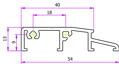
Prag TP03 Soglia TP03 Küszöb TP03
