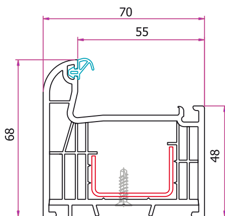
Toc ușă TP6704 - standard Telaio porta TP6704 - standard Ajtó tok A TP-6704A
