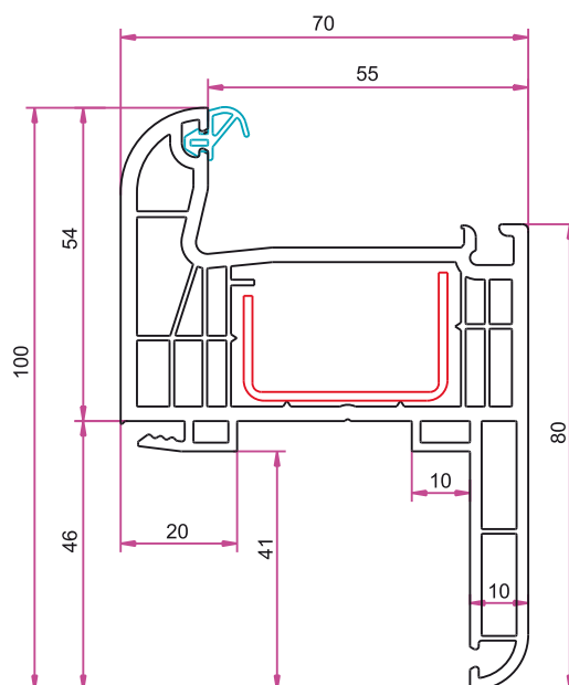
Toc Renovare TP 6705 Telaio di ristrutturazione TP6705 Felújító tok TP6705
