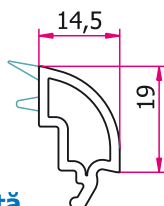
Baghetă 32 mm TP-6201 Fermavetro doppio labro 32 mm TP-6201 Üvegezőléc 32 Mm Tp-6201
