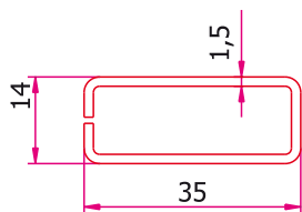
Armătură R505/15 Greutate: 1,035 kg/m Rinforzo R505/15 Peso: 1,035 kg/m Merevítés R505/15 Súly 1,035 kg/m
