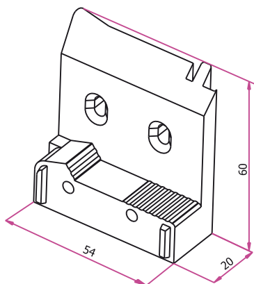
Conector prag Al TP6601 Connettore soglia Al TP6601 Küszöb Al TP6601
