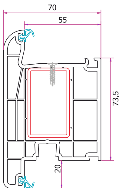
Cercevea ușă d.e. TP6702 - standard Anta porta a.e. TP6702 - standard Kifele nyíló ajtószárny A TP-6702A
