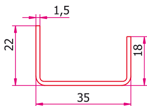
Armătură R3522/15 Greutate: 0,816 kg/m Rinforzi R3522/15 Peso: 0,816 kg/m Merevítés R3522/15 Súly 0,816 kg/m
