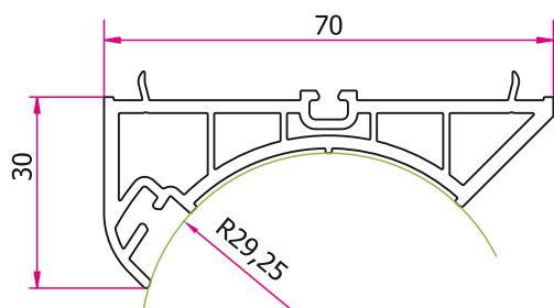
Profil cuplare TP-6306 Profilo accoppiamento TP-6306 Csősoroló csatlakozó TP-6306
