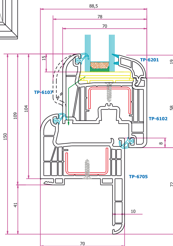
Secțiune latură inferioară Sezione lato inferiore Alsó oldal keresztmetszete
