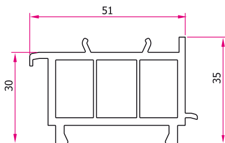
Cuplaj perete 35mm TP-5310 Accoppiatore per davanzale 35mm TP5310 Toktoldó 35mm TP5310
