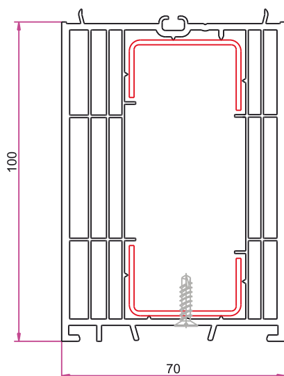
Profil adăugare 100 TP6302 Profilo agg. 100 TP-6302 Takaró 100 TP-6302
