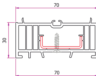
Profil de adăugare TP-6301 Profilo agg. TP-6301 Takaró TP-6301
