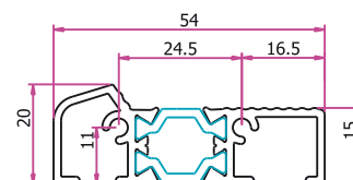
Prag Al cu bariera termica TP6510 Soglia alluminio di sbarramento termica TP6510 Alumínium küszöb (hőhidas) TP6510
