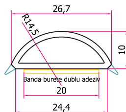
Bagheta Ornament B TP6203 Bacchetta Ornamento B TP6203 Ornament üvegezőléc B TP6203
