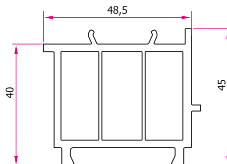
Cuplaj perete 45 mm TP-5301 Accoppiatore per davanzale 45mm TP5301 Toktoldó 45mm TP5301
