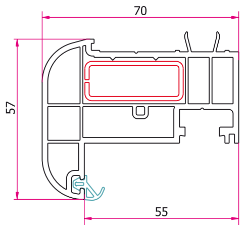
Bordură ușă TP-6104 Scambio battuta porta TP-6104 Ajtó váltószárny TP-6104
