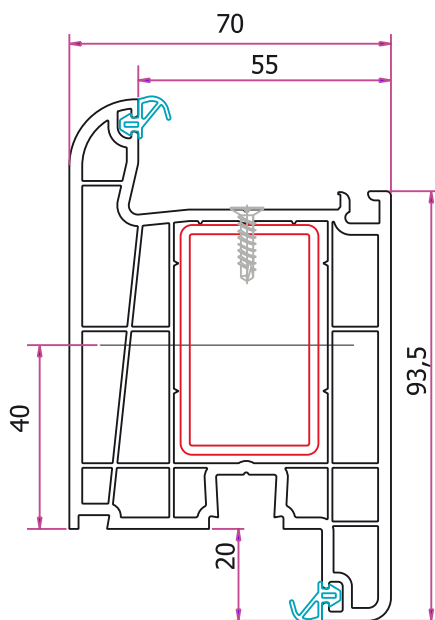
Cercevea ușă d.i. TP6701 - standard Anta porta a.i. TP6701 - standard Befele nyíló ajtószárny A TP-6701A
