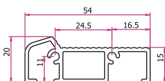
Prag Al fara bariera termica TP6511 Soglia alluminio senza sbarramento termica TP6511 Alumínium küszöb (hőhídmentes) TP6511
