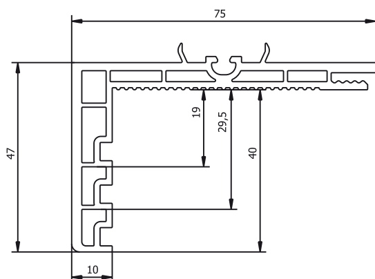
Profil renovare TP5404 Profilo ristrutturazione TP5404 Felújító profil TP5404
