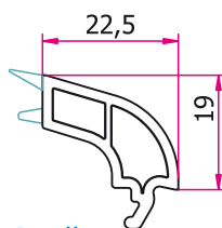
Baghetă 24 mm TP-6202 Fermavetro doppio labro 24 mm TP-6202 Üvegezőléc 24 Mm Tp-6202
