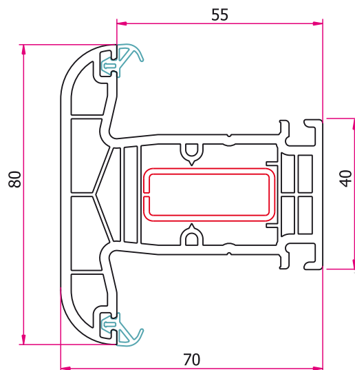
Montant TP6103 - standard Montant TP6103 - Eco Montante TP6103 - standard Montante TP6103 - Eco Osztó TP6103 - standard Osztó TP6103 - Eco
